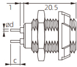
印制板 (Print)
